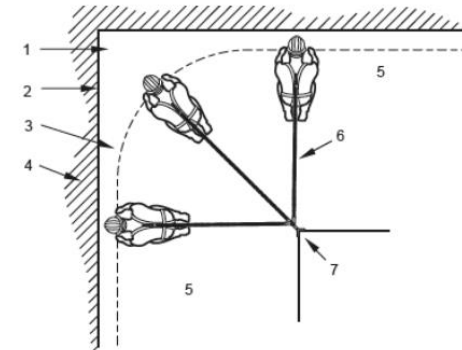
a) Sistema de restrição que impede o usuário de alcançar o canto do telhado
